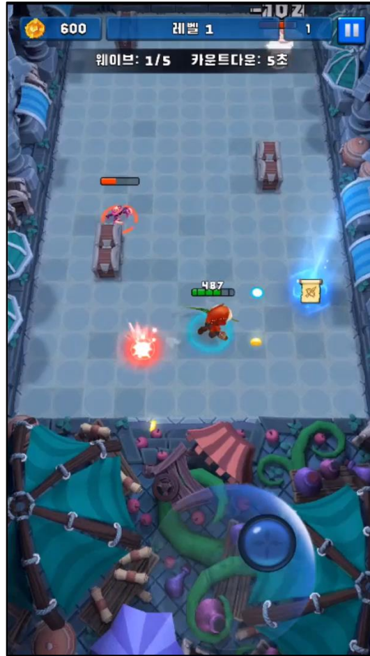
<원본 앱>
