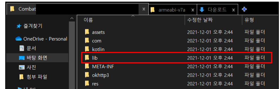
<변조 앱>
