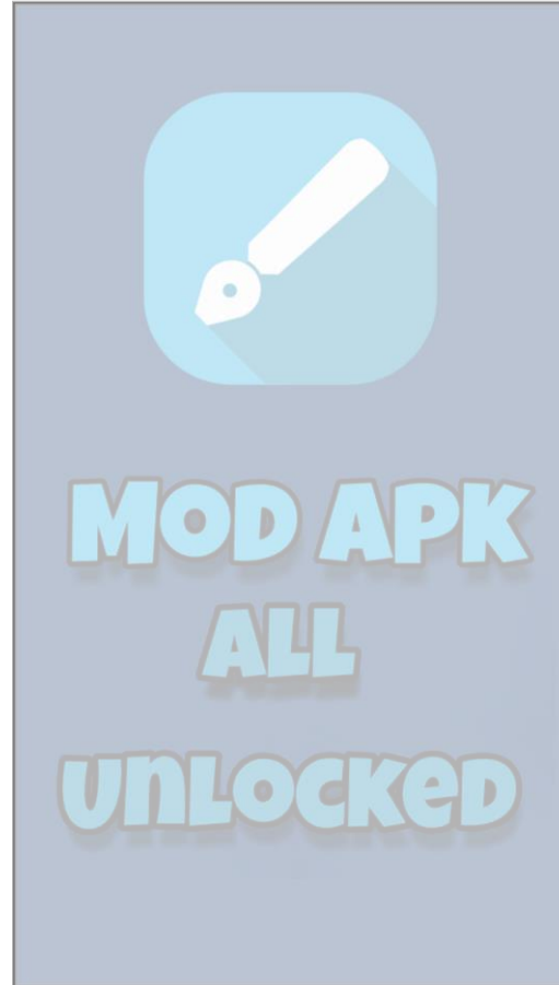
〈인증 우회〉
