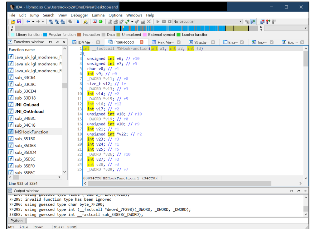
〈MSHookFunction〉
