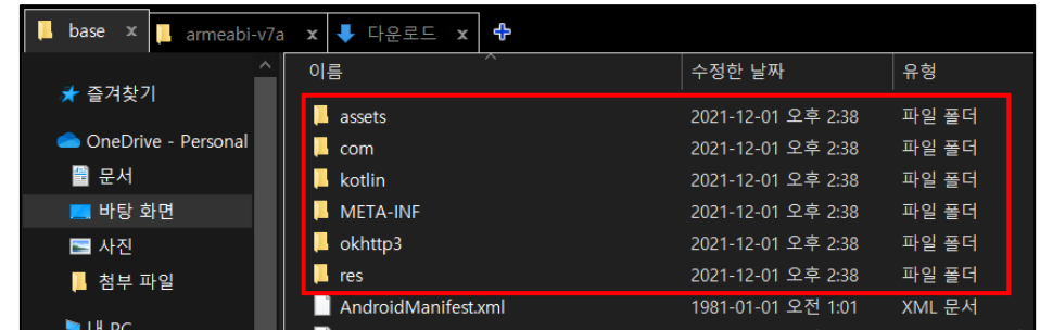
<원본 앱>
